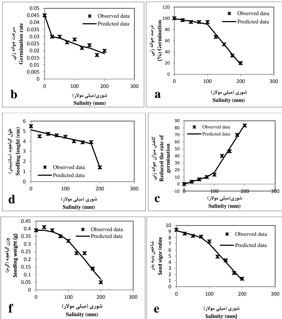
شکل ۱- روند تغییرات درصد جوانه‌زنی (a)، سرعت جوانه‌زنی (b)، کاهش میزان جوانه‌زنی (c)، طول گیاهچه (d)، شاخص بیه بدر (e) و وزن گیاهچه (f) در سطوح مختلف شوری در گیاه نوروبک.
